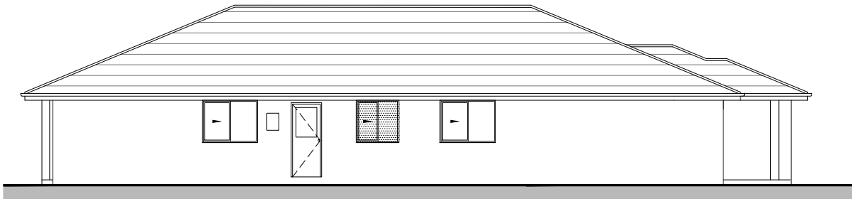
Elevation 3
